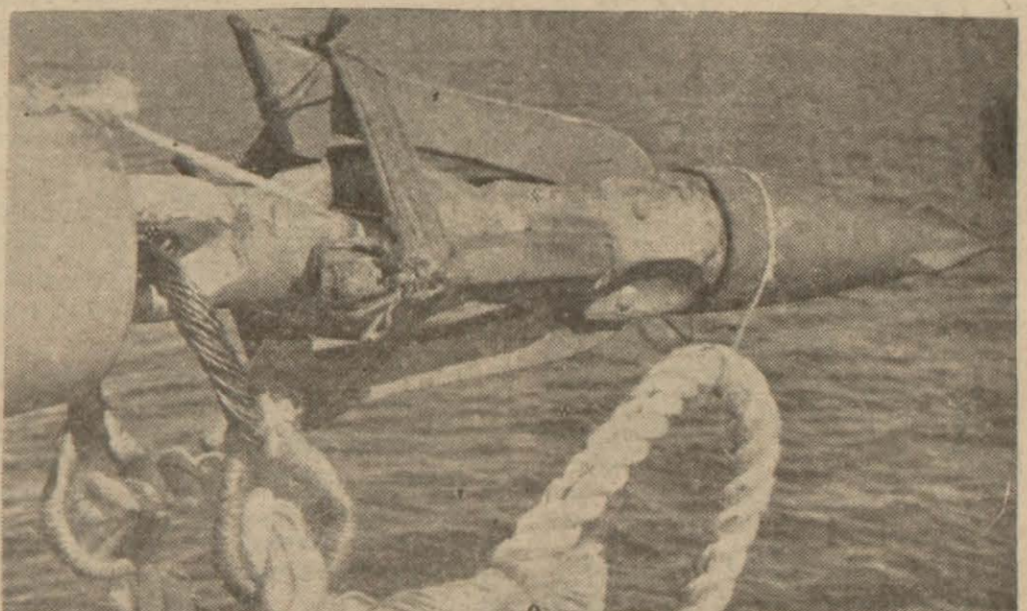
Modern balina avı gemilerinde zıpkın atan top bu şekildedir
